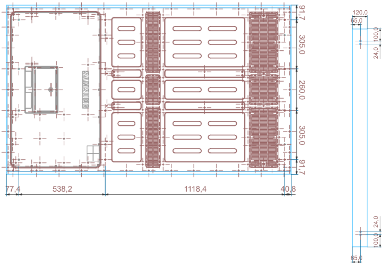
Outdoor TFT 75" – Vue arrière et latérale
