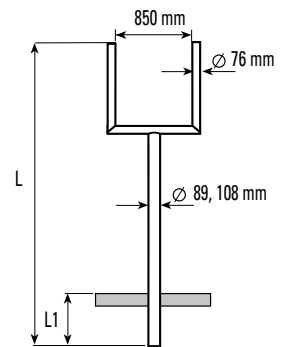
RM108/76/2/3600 (L = 3600, L1 = 600) Rohrmast für 2 Spiegel VS-A8010R, oben geschlossen Mât tubulaire pour 2 miroirs VS-A8010R, fermé en haut
