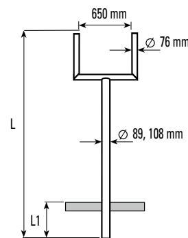
RM89/76/2/3600B (L = 3600, L1 = 600) Rohrmast für 2 Spiegel VS-A6080R, oben geschlossen Mât tubulaire pour 2 miroirs VS-A6080R, fermé en haut
