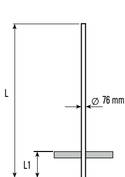
RM76/3600 (L = 3600, L1 = 600) RM83/3600 (L = 3600, L1 = 600) Rohrmast für 1 Spiegel, oben geschlossen Mât tubulaire pour 1 miroir, fermé en haut
