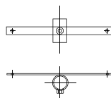
BKL40 ... (b=400/500/560/600/750/840/1000) Einseitige Befestigungen für mobile Signale, geschraubt, feuerverzinkt, zum Festklemmen auf 1"-Rohr Fixations unilatérales pour signaux mobiles, fermeture à vis, galvanisées, pour fixation sur mât tubulaire 1"
