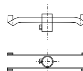
BB40/2 (Normalformat/format normal) BB120/2 (Grossformat/grand format) Doppelseitige Befestigungen für mobile Signale, feuerverzinkt, pro Tafel 2 Stk. zum Festklemmen auf 1"-Rohr Fixations bifaces pour signaux mobiles, galvanisées, 2 pces par panneau pour fixation sur mât tubulaire 1"
