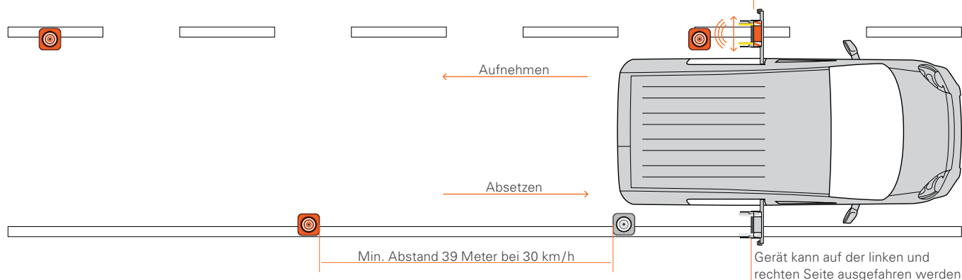
Beweglicher Kopf, ausgestattet mit einem Sensor. Zum präzisen Absetzen und Aufnehmen der Kegel.
