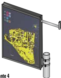
Variante 4 Panel als Fahnen- und Wandmontage mit verschiedenen seitlichen Befestigungsmöglichkeiten Panneau comme montage en drapeau ou mural avec diverses possibilités de fixation latérale, Profil Alu largeur = 50 mm
