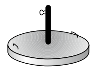
BE67 (Ø 670 mm, 50 kg) BE80 (Ø 800 mm, 80 kg) Betonsockel mit Flacheisen verstärkt, mit feuerverzinktem Rohrstützen für 1"-Rohr. Mit 2 Handgriffen Socle en béton rond, renforcé par anneau fer plat, avec tubulure galvanisée pour mât tubulaire 1". Avec 2 poignées
