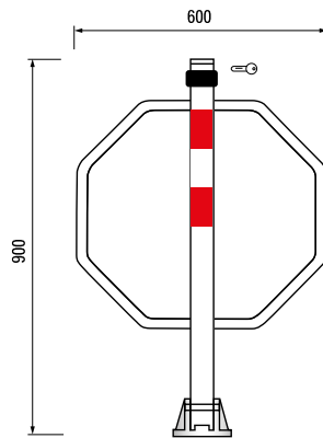
PAP96 Version mit seitlichem Bügel
