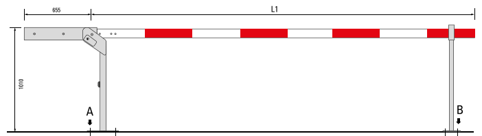
HSA (mit Aufleger) Handschranke mit retroreflektierendem Alu-Schrankenbaum, mit Schrankenständer inkl. Bodenplatte
